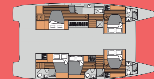
MAESTRO 5 CABINS
